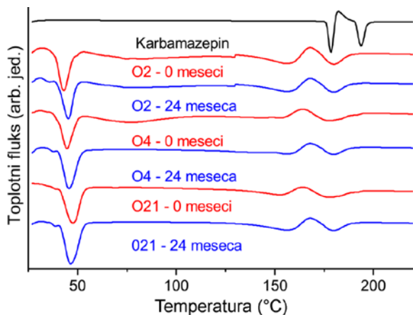
Slika 5. DSC krive karbamazepina i ispitivanih uzoraka O2, O4 i O21 nakon izrade i nakon 24 meseca
