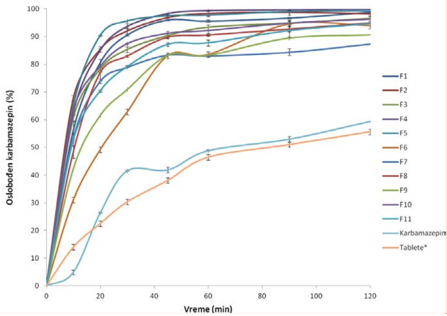
Slika S2. Profili brzine rastvaranja karbamazepina iz izrađenih čvrstih disperzija, praška karbamazepina i tableta karbamazepina sa trenutnim oslobađanjem Figure S2. Dissolution profile of carbamazepine prepared from solid dispersion, carbamazepine powder and carbamazepine tablets with immediate release
