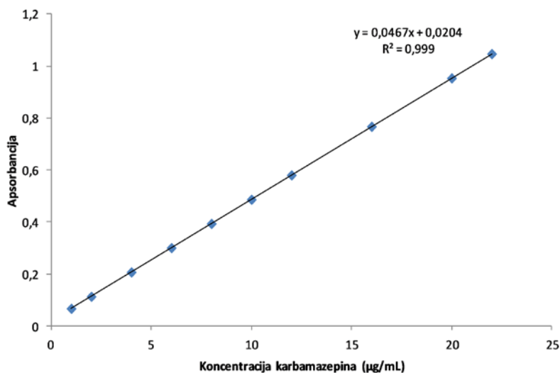
Slika S1. Kalibraciona kriva za UV-spektrofotometrijsko određivanje karbamazepina Figure S1. Calibration curve for UV-spectrophotometric determination of carbamazepine
